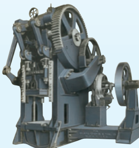
創立時、当社が初めて導入したプレス機 (600tトッフルドローイングプレス機)
